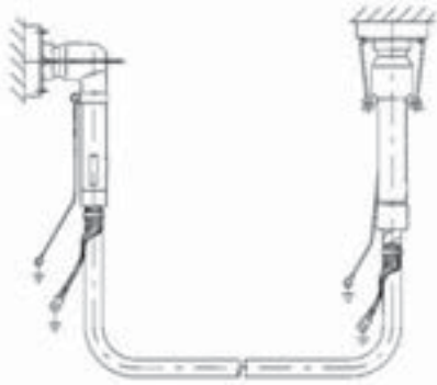
Verbindung zwischen Schaltanlage und Transformator mit 250A Durchführungen: Connection between switchgear and transformer with 250A bushings:
