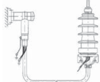
Verbindung zwischen Transformator und Endverschluss mit Stützerfunktion (z. B. Einsatz in Schnellzügen der Deutschen Bahn AG): Connection between transformer and termination with support function (e. g. installed in express trains of Deutsche Bahn AG):
