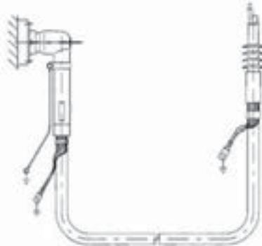
Verbindung zwischen Schaltanlage und Transformator mit Isolatorenanschluss: Connection between switchgear and transformer with insulators:
